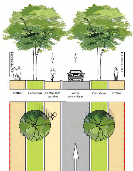
Profil en travers à valeur indicative
