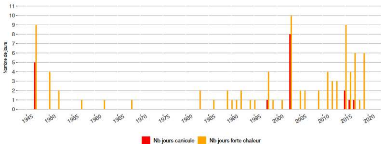
Figure 10: Évolution du nombre de jours de canicule et de forte chaleur à Clermont-Ferrand (1947-2019 – altitude 331 m) [source : site internet ORCAE]
