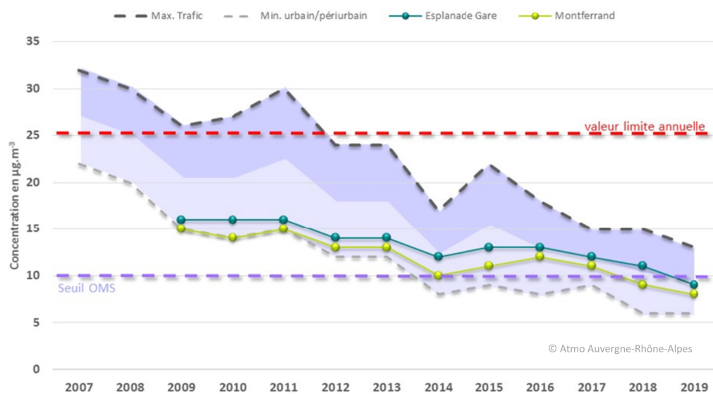
Figure 42: Historique des moyennes annuelles en PM 2,5 en situation de fond et de proximité dans la zone d'étude [Source : Atmo AuRA]
