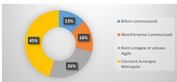
Figure 85: Emissions respectives de PM 10 des EPCI du Grand Clermont en 2019
