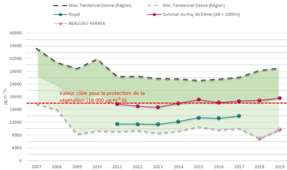
Figure 44: Evolution de l'AOT 40 en situation de fond périurbain/rural [Source : Atmo AuRA]
