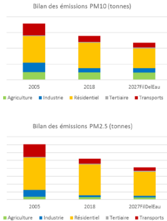
Figure 54 : Origine sectorielle des particules fines [Source : Atmo AuRA]
