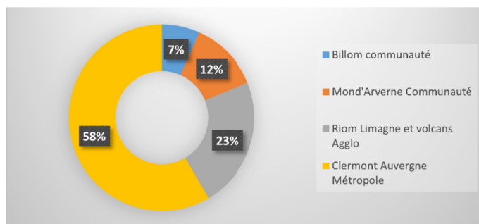
Figure 83: Emissions respectives de NO x des EPCI du Grand Clermont en 2019
