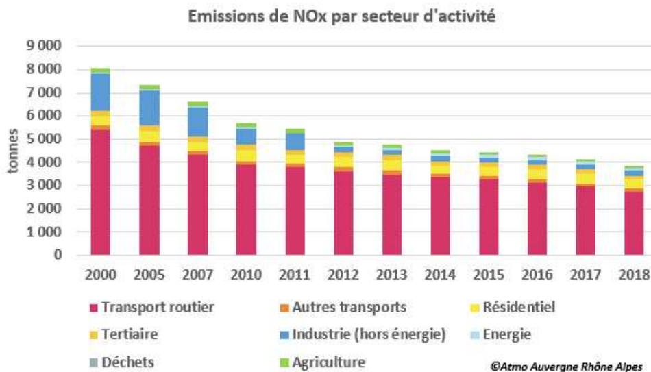
Figure 48 : Evolution des émissions de NO x par secteur sur le périmètre d'étude du PPA [Source : Atmo AuRA]
