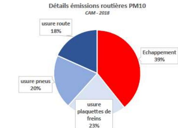
Figure 55 : Détail des émissions routières des PM_{10} sur le territoire de CAM en 2018 [source : Atmo AuRA]
