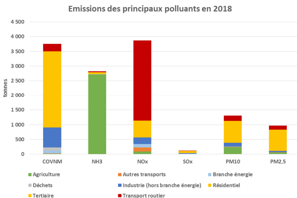
Figure 53: Répartition des émissions par secteur d'activité [Source : Atmo AuRA, inventaire ESPACE V2020]
