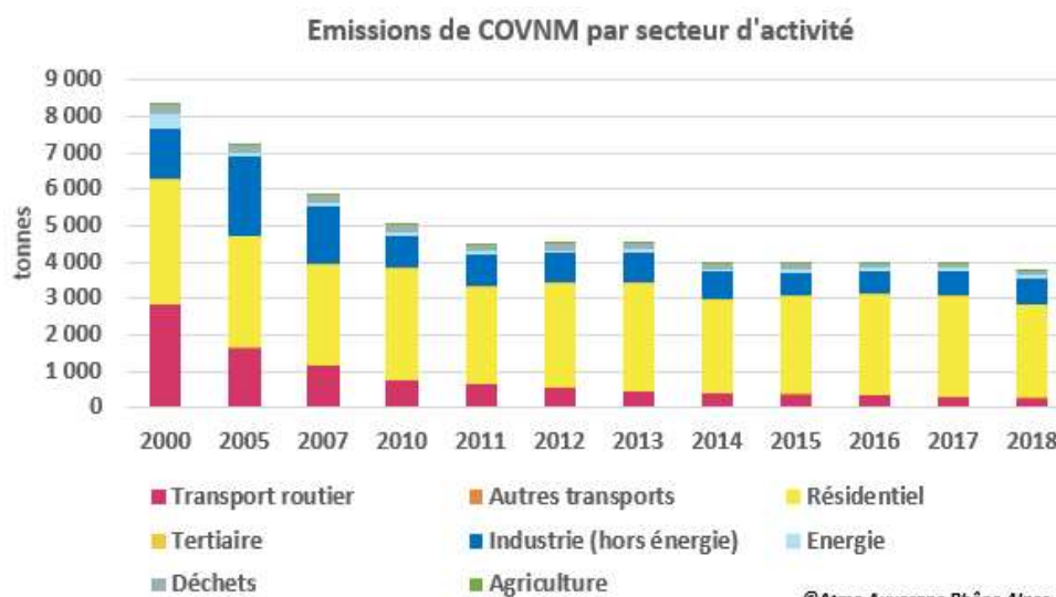
Figure 50 : Evolution des émissions de COVNM par secteur sur le périmètre d'étude [Source : Atmo AuRA]
