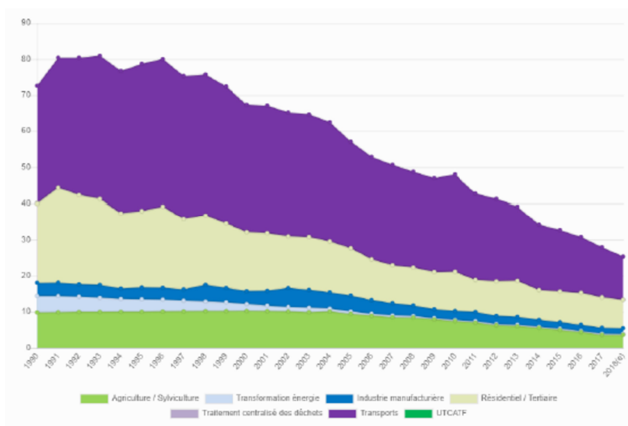
Figure 34 : Evolution des émissions de « Black Carbon » de 1990 à 2017 en France [source : CITEPA]
