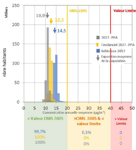
Figure 91 : Scénario PPA – Histogramme de distribution de l'exposition de la population au \text{PM}_{10}
