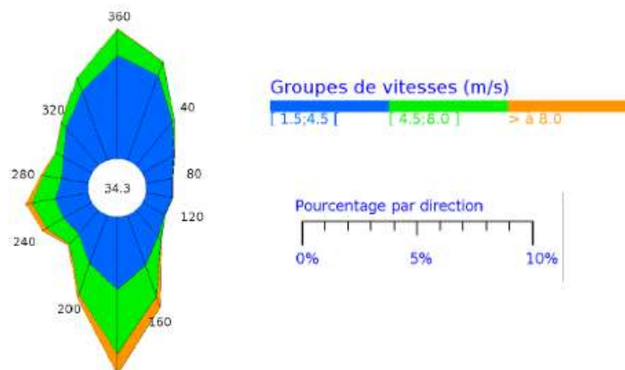
Figure 11: Fréquence des vents en fonction de leur provenance en % [Source : Météo France]
