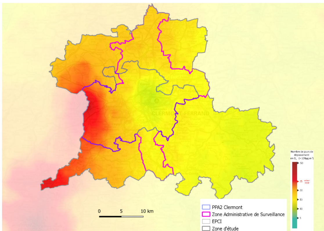
Figure 64: Nombre de jours de dépassements de la valeur cible pour l'O 3 en 2019 [Source : Atmo AuRA]
