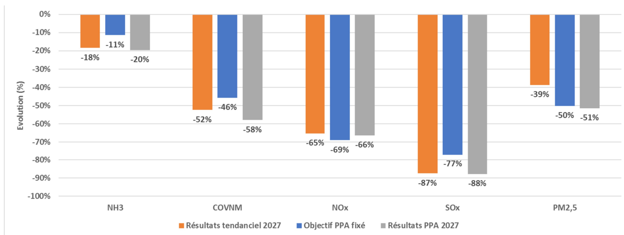
Figure 88 : Comparaison des projections de baisse d'émissions aux objectifs de réduction sur le périmètre du PPA [source : Atmo AuRA]
