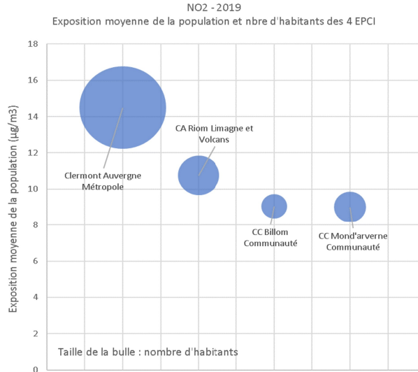
Figure 66: Exposition moyenne de la population au NO 2 par EPCI en 2019, en µg/m 3 [Source : Atmo AuRA]
