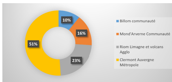
Figure 84: Emissions respectives de PM 2,5 des EPCI du Grand Clermont en 2019
