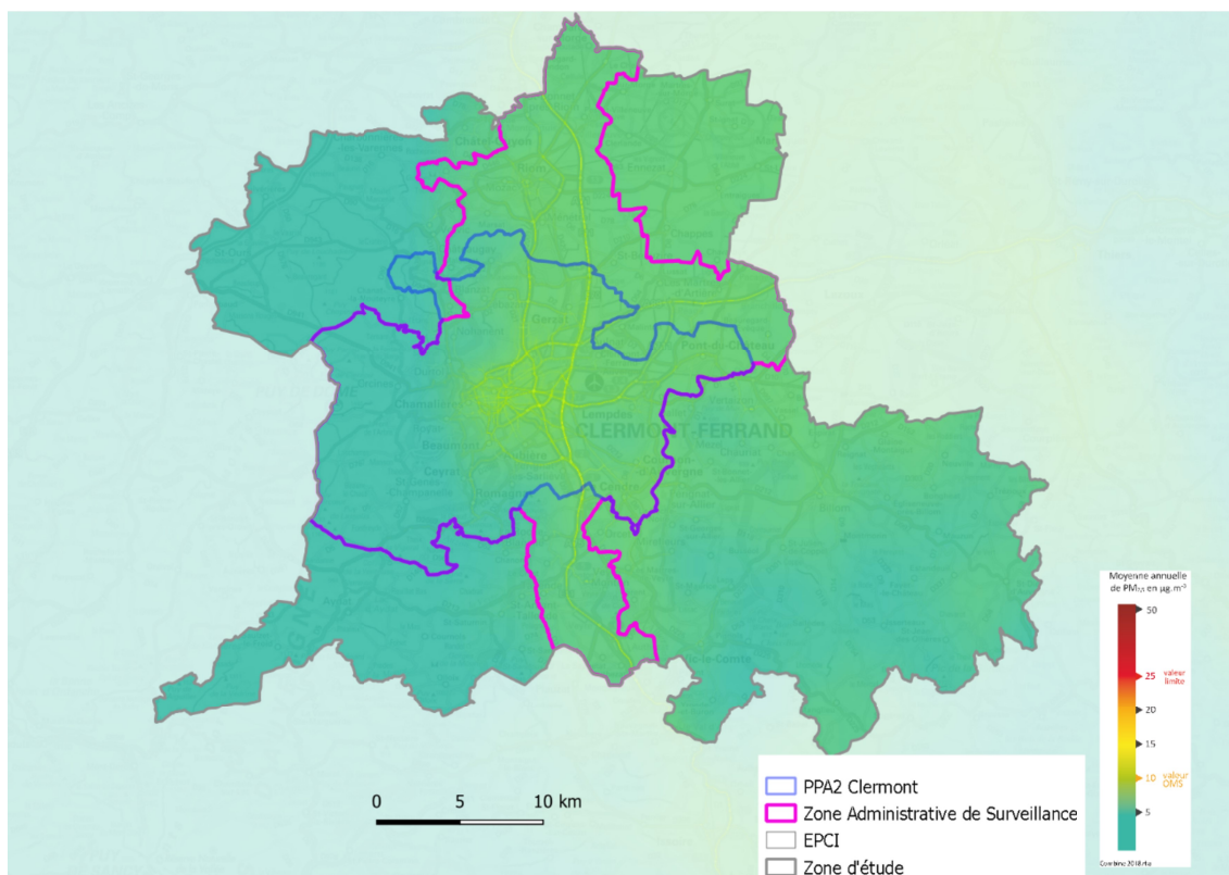
Figure 63: Concentrations annuelles en PM_{2,5} en 2019 [Source : Atmo AURA]
