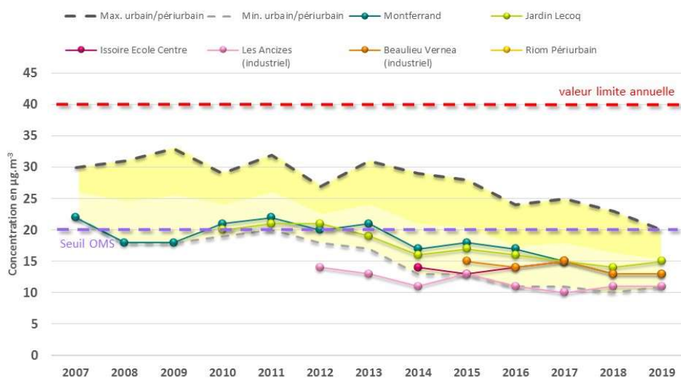
Figure 41: Historique des moyennes annuelles en PM 10 en situation de fond dans la zone d'étude [Source : Atmo AuRA]
