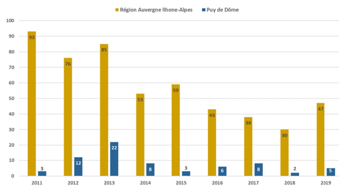
Figure 46: Épisodes de pollution : historique des vigilances de 2011 à 2019 en AuRA et Puy-de-Dôme
