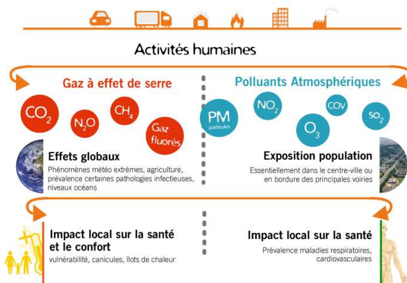
Figure 5: GES et polluants atmosphériques : sources, effets et impacts. [Source : Atmo AuRA]
