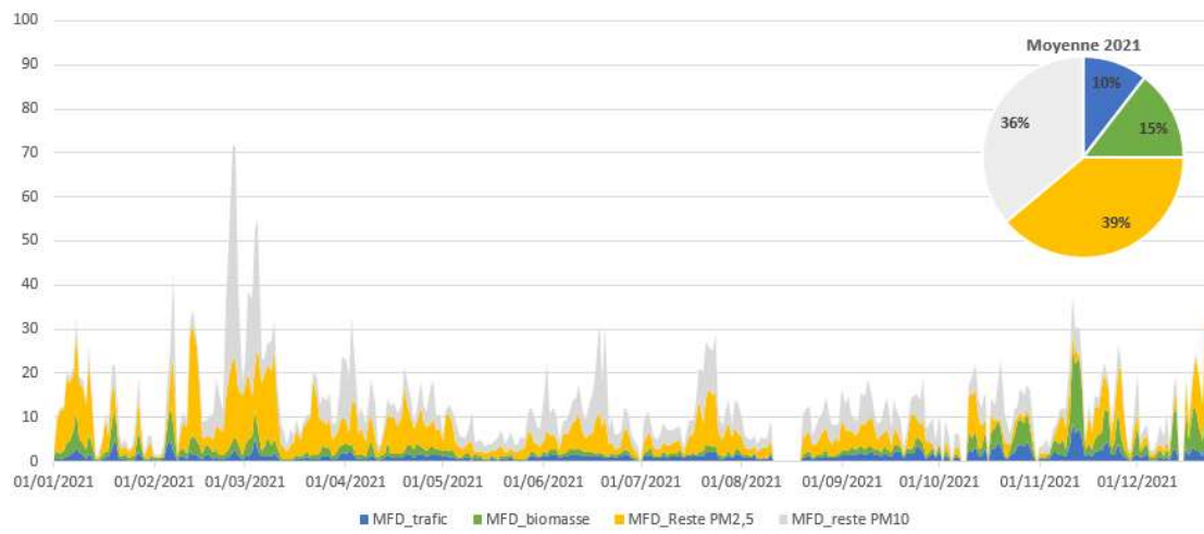
Figure 37 : contribution en masse des PM_1 aux PM_{10} et apports relatifs des combustions de biomasse et carburant dans les PM_1 [Source : Atmo AuRA]
