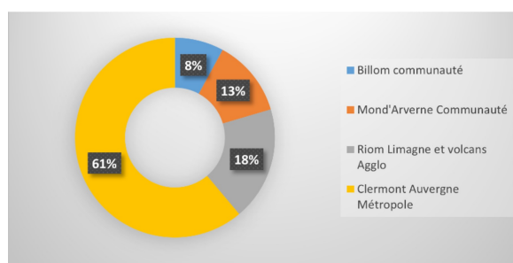
Figure 87: Emissions respectives de COVNM des EPCI du Grand Clermont
