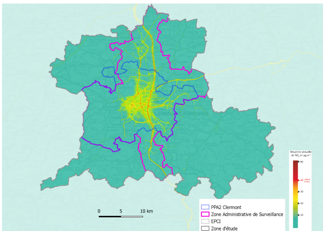
Figure 61: Concentrations annuelles en NO 2 en 2019 [Source : Atmo AuRA]
